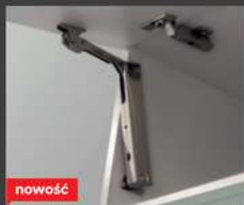
Szafki wiszące ...WOX... wyposażone w podnośnik z regulacją mocy.
